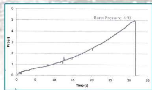
نمودار روند افزایش فشار در نمونه تست های بازرسی
